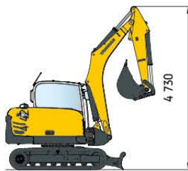
Abb. 1: Arbeitseinrichtung
