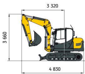
Abb. 1: Arbeitseinrichtung
