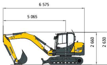
Abb. 2: Transportstellung
